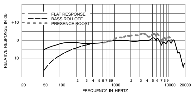
RÉPONSE EN FRÉQUENCE TYPIQUE FIGURE 4
