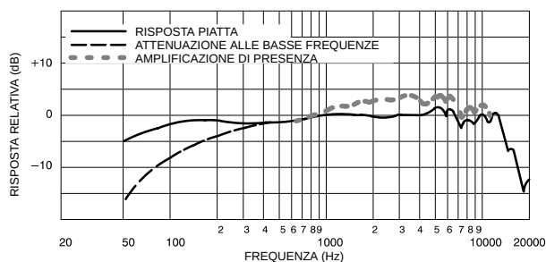
RISPOSTA IN FREQUENZA TIPICA
