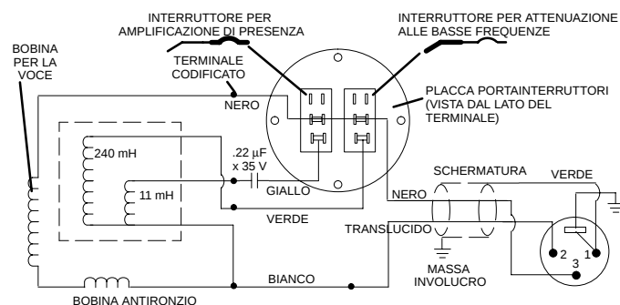
CONNESSIONI INTERNE
