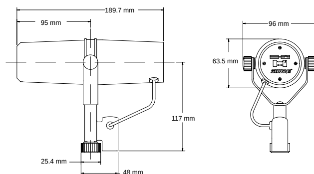
DIMENSIONI COMPLESSIVE
