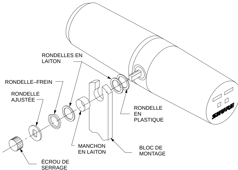
MONTURE – VUE ÉCLATÉE FIGURE 3
