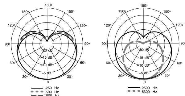
DIAGRAMMI POLARI TIPICI
