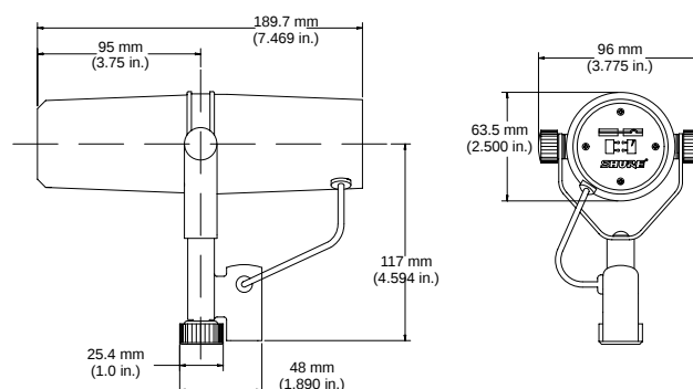
DIMENSIONS HORS TOUT FIGURE 6
