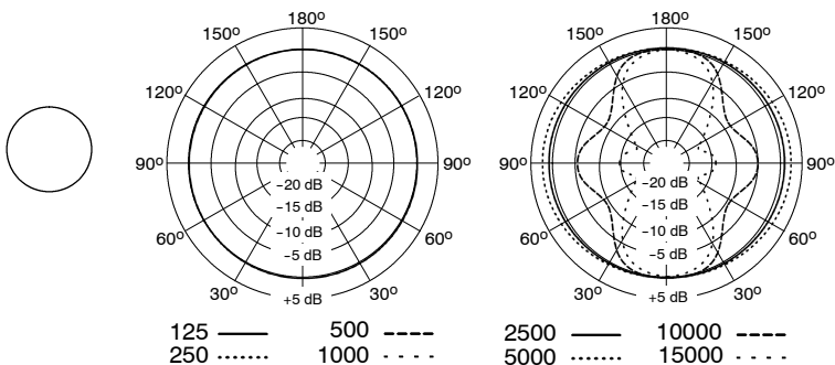
FIGURA 6. DIAGRAMMI POLARI TIPICI
