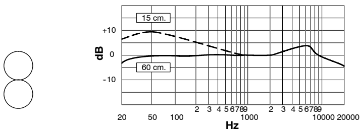
FIGURA 7. RISPOSTA IN FREQUENZA TIPICA
