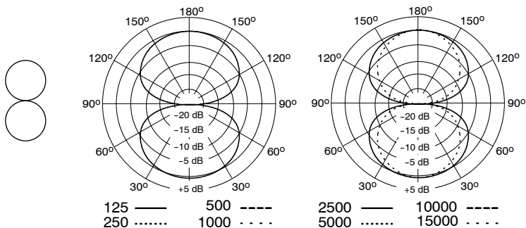
FIGURA 8. DIAGRAMMI POLARI TIPICI
