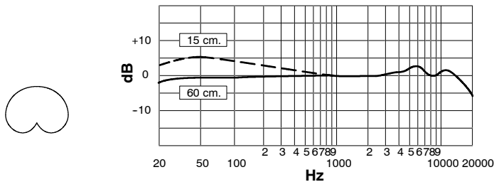
FIGURA 3. RISPOSTA IN FREQUENZA TIPICA
