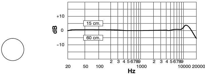
FIGURA 5. RISPOSTA IN FREQUENZA TIPICA
