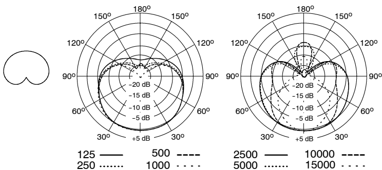
FIGURA 4. DIAGRAMMI POLARI TIPICI
