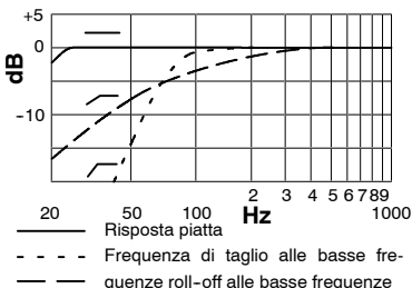
Figura 2. Risposte alle basse frequenze
